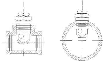
装在管接头,T型接头,连接器上
